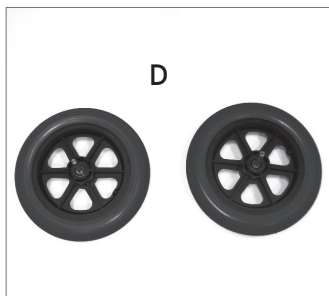
D - Petites roues arrière (diamètre 30 cm) modèle transit
